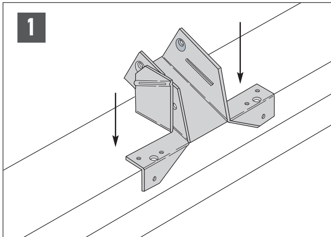
1 Posicione el conector sobre la placa superior.
