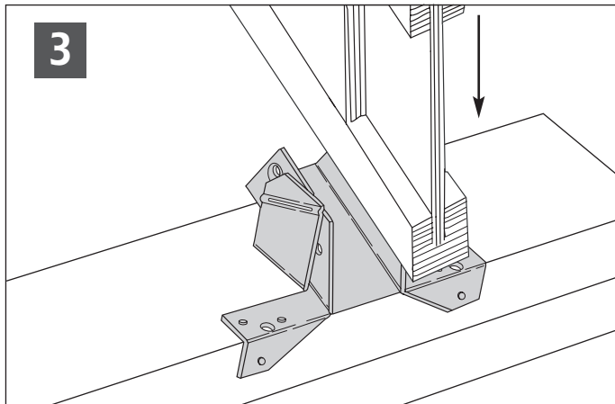
3 Inserte el cable en el hueco para el mismo. Ejerza presión hacia abajo para asentar totalmente el cable.
