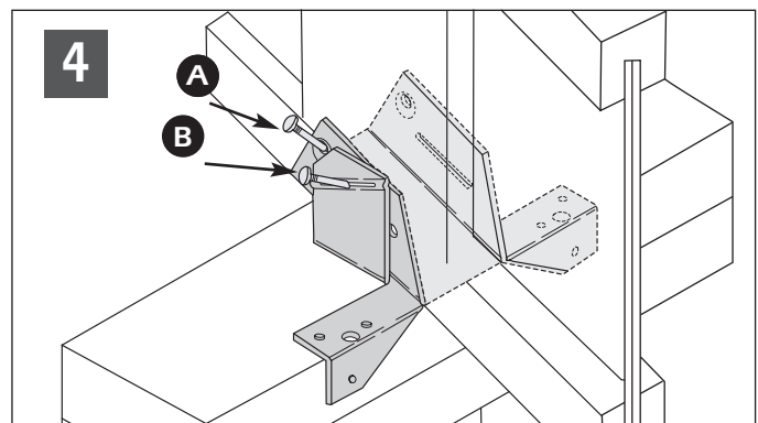
4 Sujete el cable al conector con (4) clavos 10d x 1-1/2" pulg. en el hueco del mismo; (A) - 2 instalados en un ángulo descendente a través de guías de claveteado con hendiduras y (B) - 2 instalados a través de ranuras opuestas.
