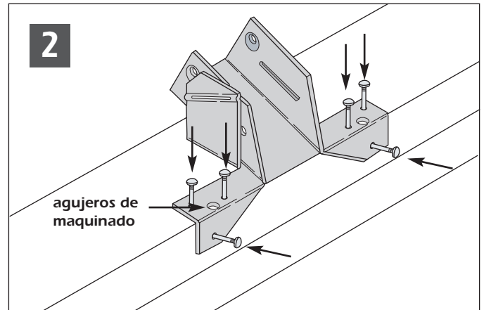
2 Sujete el conector al lado exterior de la placa superior con (6) clavos 10d. No instale los clavos a través de grandes agujeros de maquinado.
