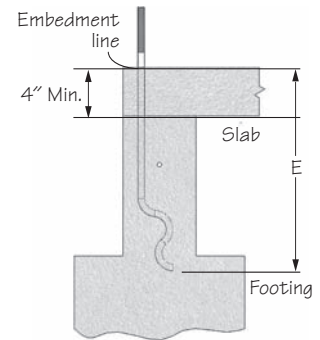
Typical double pour installation
